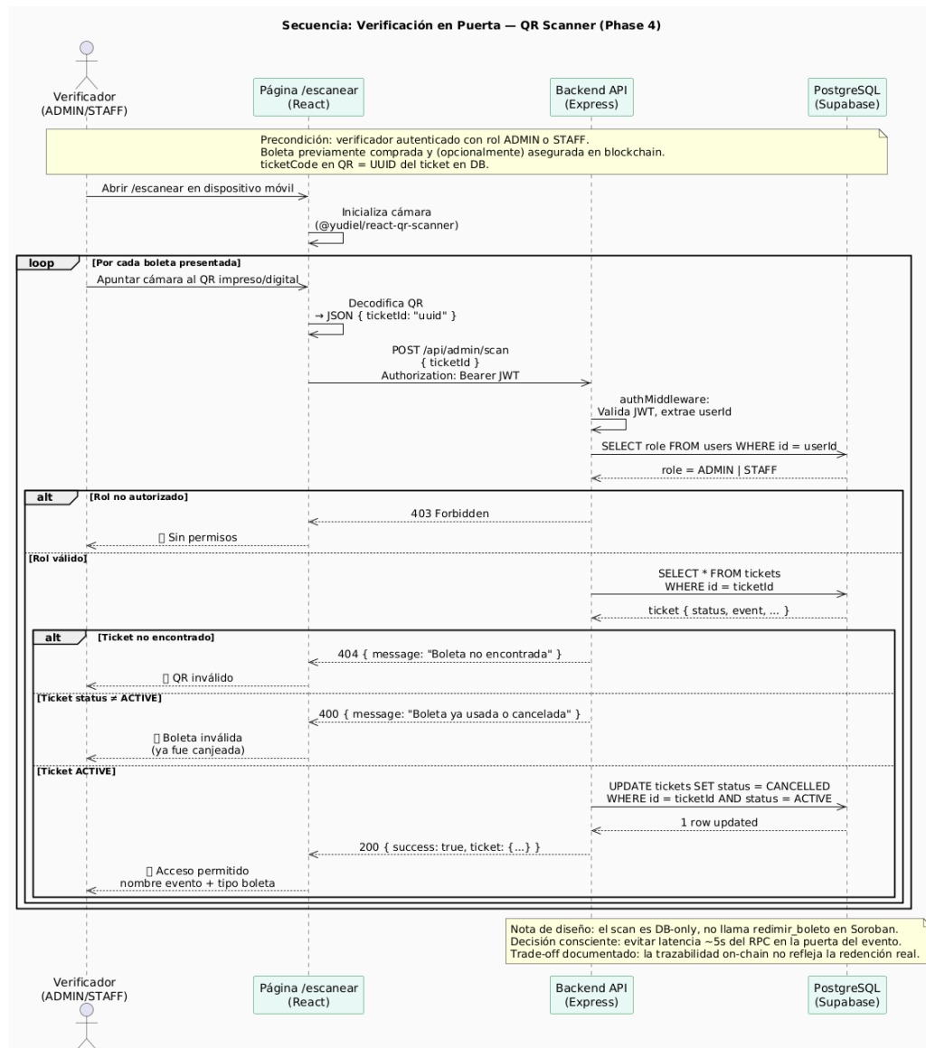
Figura 5: Diagrama de secuencia – Verificación en puerta con escáner QR (Phase 4)
